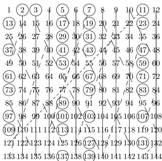
Figura 5.1: Il crivello di Eratostene.
