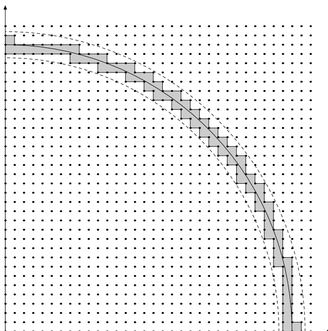
Figura 2.2: Dimostrazione del Teorema di Gauss 2.2.2.
