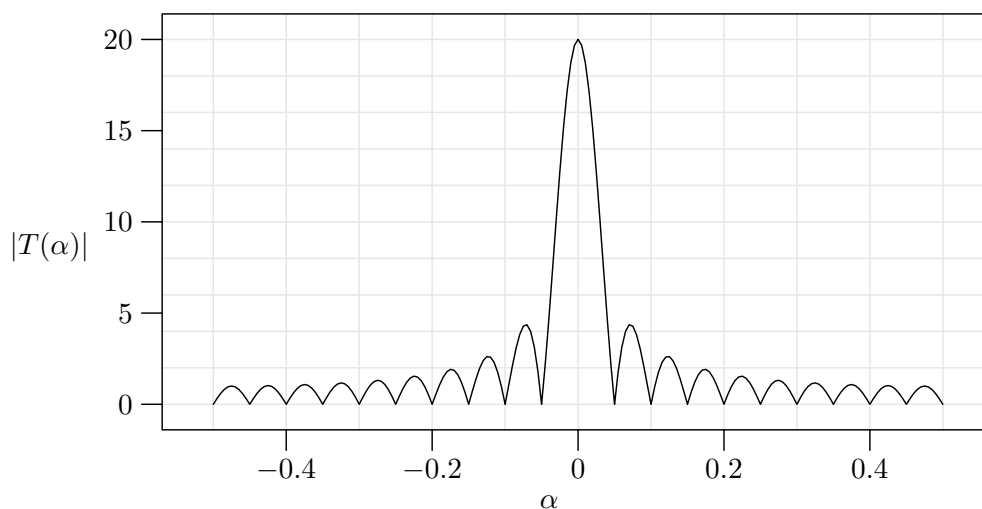
Figura 7.2: Il grafico della funzione |T_{20}(\alpha)| nel quale si nota molto bene che questa funzione ha un grosso picco in prossimità dei valori interi di \alpha , ed è altrimenti molto piccola.
