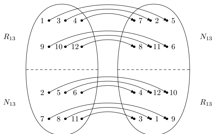
Figura 1.3: Dimostrazione dell'ultima parte del Lemma 1.6.3 per p = 13 ed a = 5 .
