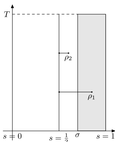
Figura 6.5: Come usare la formula (6.10.4).
