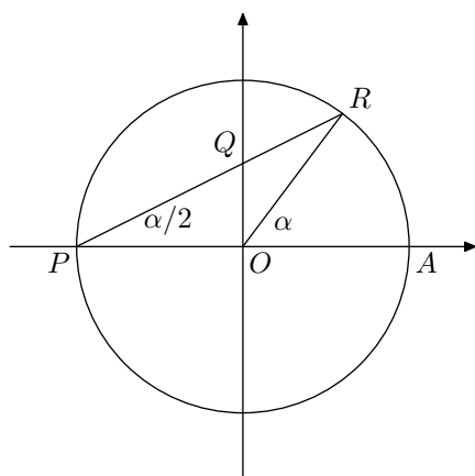
Figura 1.2: Come parametrizzare i punti della circonferenza unitaria.
