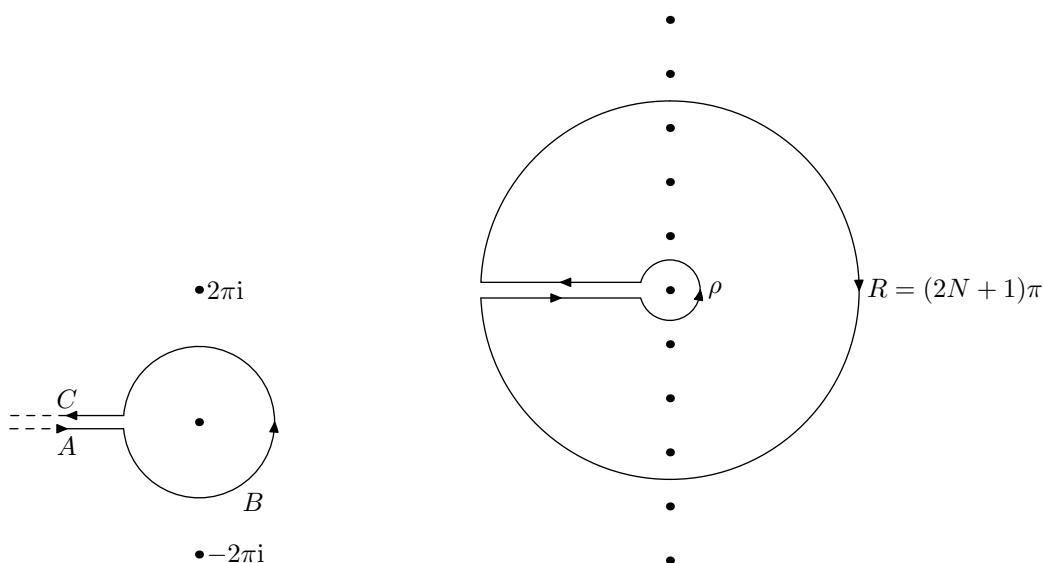
Figura 6.1: I cammini di integrazione nel Teorema 6.2.4.
