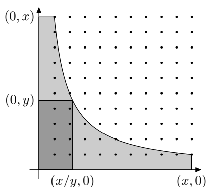
Figura 2.1: Dimostrazione del Teorema 2.1.13.
