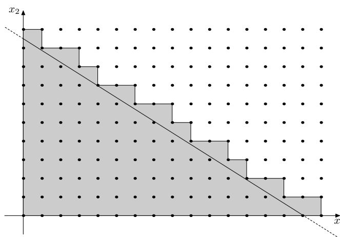
Figura 1.4: La dimostrazione del Teorema di Schur 1.7.2 nel caso in cui k = 2 e \mathfrak{P}_f = \{2, 3\} . L'area in grigio è uguale a |V(x)| .
