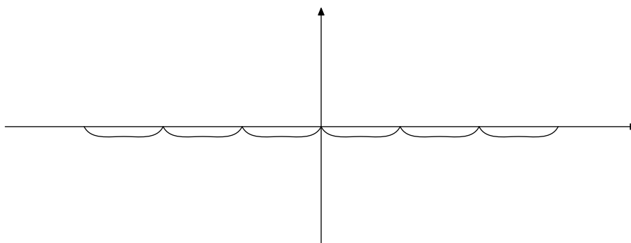
Figura A.2: Il grafico della funzione g(t) := \frac{1}{2}(\{t\}^2 - \{t\})
