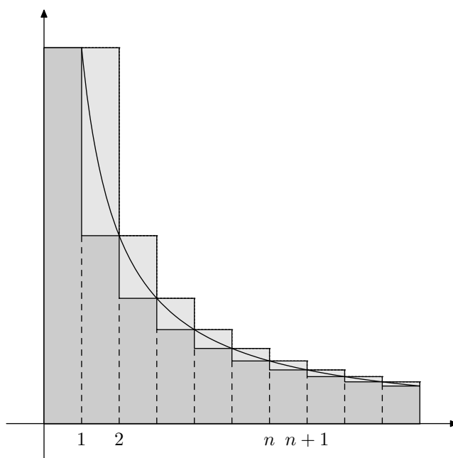
Figura A.1: Dimostrazione del Lemma A.1.3: l'area in grigio chiaro non supera f(1) . L'area in grigio scuro fra x = 0 ed x = n è piú grande di f(1) + \dots + f(n) .
