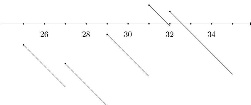
Figura 3.3: Il grafico di \psi(x) - x per x \in [25, 35] . Il grafico di V(\xi) si può ricavare da questo mediante un cambiamento di variabile, ma il comportamento qualitativo evidentemente è lo stesso.
