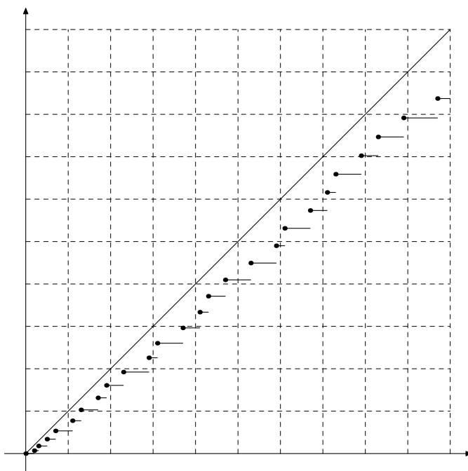
Figura 3.2: Il grafico di \theta(x) e di x per x \in [0, 100] .
