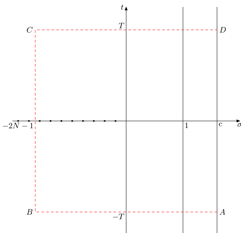
Figura 6.4: Il cammino di integrazione che si usa per dimostrare la forma troncata della formula esplicita. I tratti orizzontali del cammino deformato devono evitare gli zeri di \zeta in 0 < \sigma < 1 , mentre il tratto verticale deve evitare gli zeri banali s = -2n , indicati sull'asse reale negativo, e quindi è possibile scegliere un segmento della retta \sigma = -2N - 1 . In un secondo tempo si fa tendere N a +\infty .
