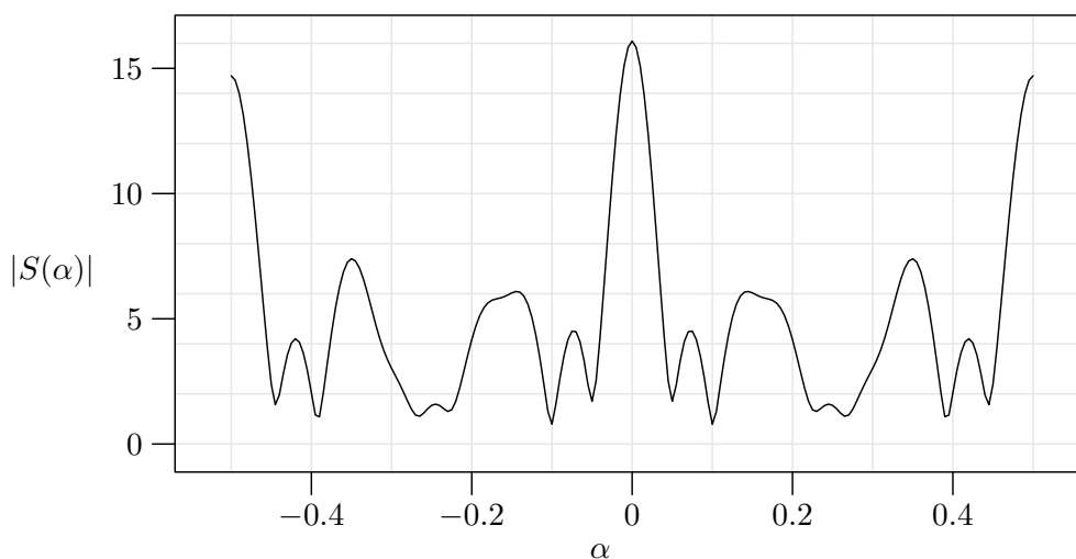
Figura 7.1: Il grafico della funzione |S_{20}(\alpha)| nel quale si notano molto bene i picchi in prossimità dei valori razionali di \alpha = 0, \frac{1}{2}, \frac{1}{3}, \frac{2}{3}, \frac{1}{6}, \frac{5}{6} , mentre in \alpha = \frac{1}{4}, \frac{3}{4} non c'è picco poiché \mu(4) = 0 .
