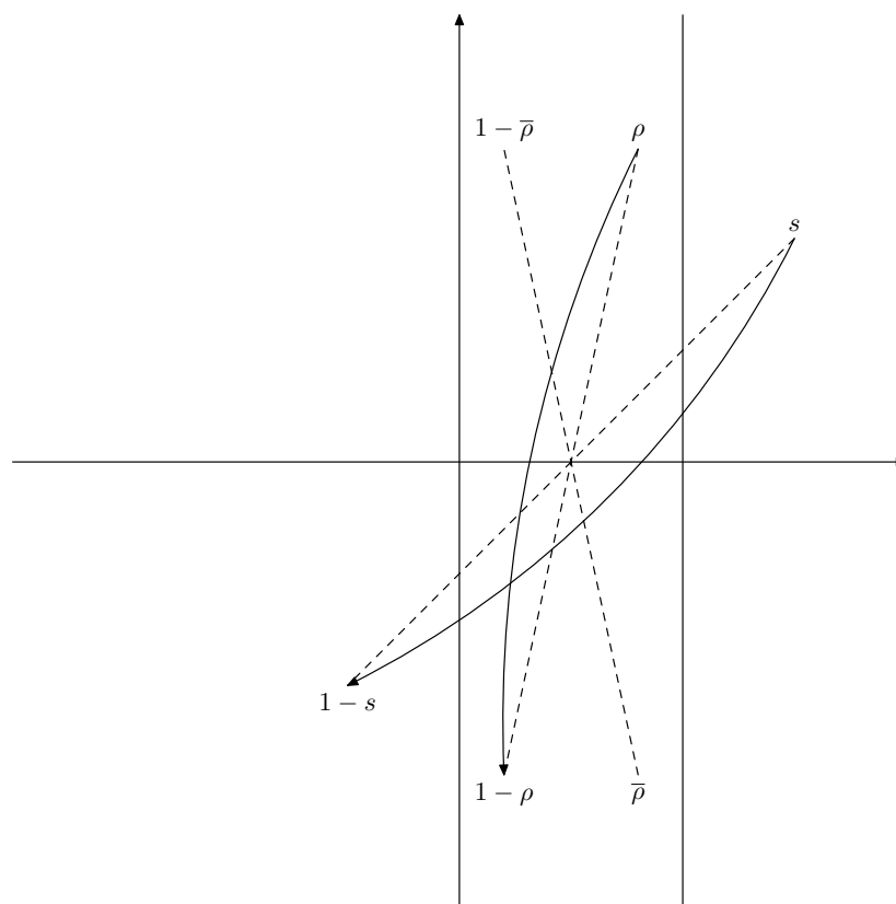
Figura 6.2: Conseguenze dell'equazione funzionale.
