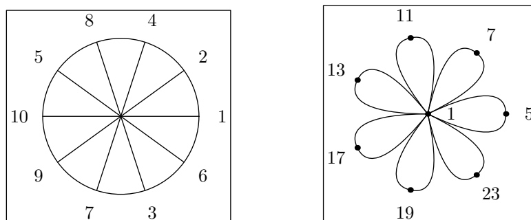
Figura 1.1: Struttura di \mathbb{Z}_{11}^* e di \mathbb{Z}_{24}^* . Gli archi connettono le potenze successive dello stesso elemento: nel caso a sinistra le potenze di 2 (che è un generatore di \mathbb{Z}_{11}^* ), nel caso a destra, poiché ogni elemento di \mathbb{Z}_{24}^* soddisfa x^2 \equiv 1 \pmod{24} , le potenze successive di x \neq 1 sono 1, x, 1, x, \dots
